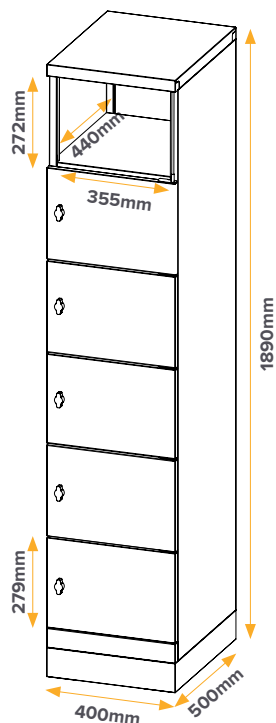
6 Door Locker
