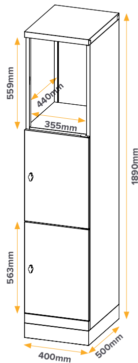
3 Door Locker
