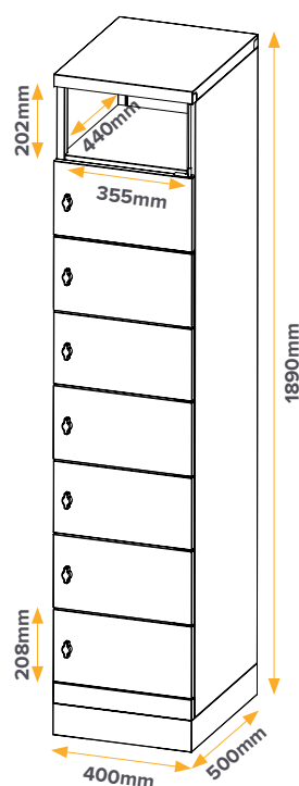
8 Door Locker
