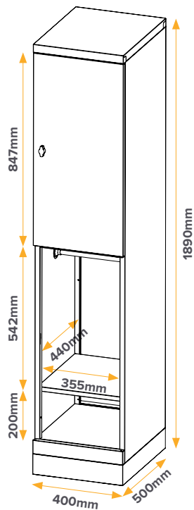
2 Door Locker
