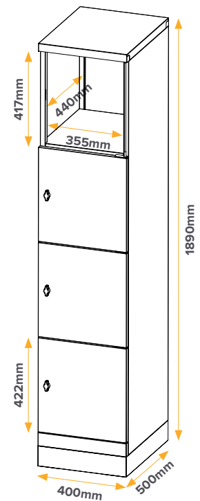
4 Door Locker
