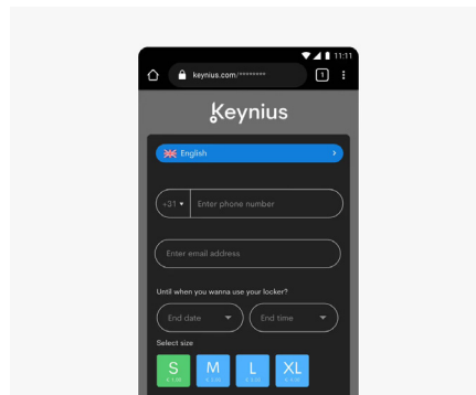
Web App
